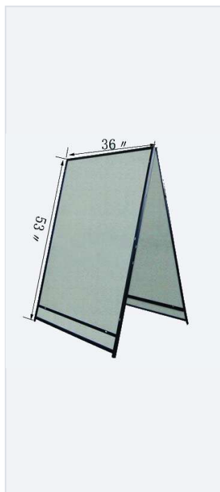
SZJ3653 A-frame · 36" × 53"
