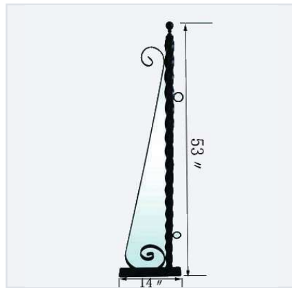
DZJ-53 20 Scroll bracket stand · 53" × 14"
