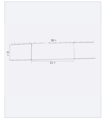
TS-D Wire step stake · 35" × 12"
